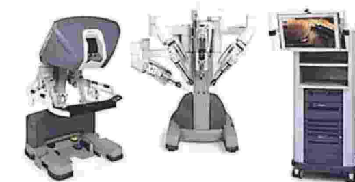
Robot DaVinci per la chirurgia robotica: 1. Consolle Chirurgica. 2. Carrello Paziente progettato per reggere gli strumenti endoscopici. 3. Carrello Visione
